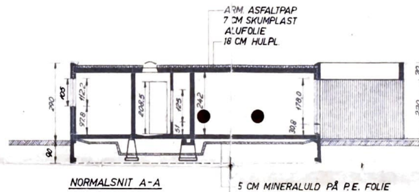
NORMALSNIT A-A
