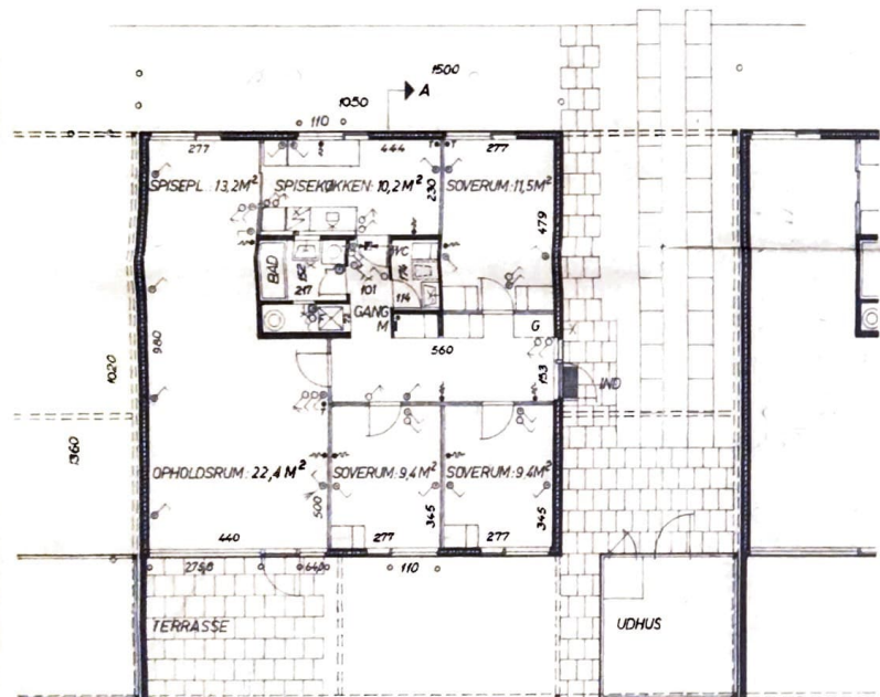
PLAN 1:100
